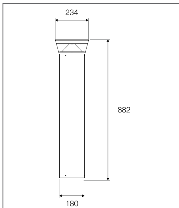
Dimensions
